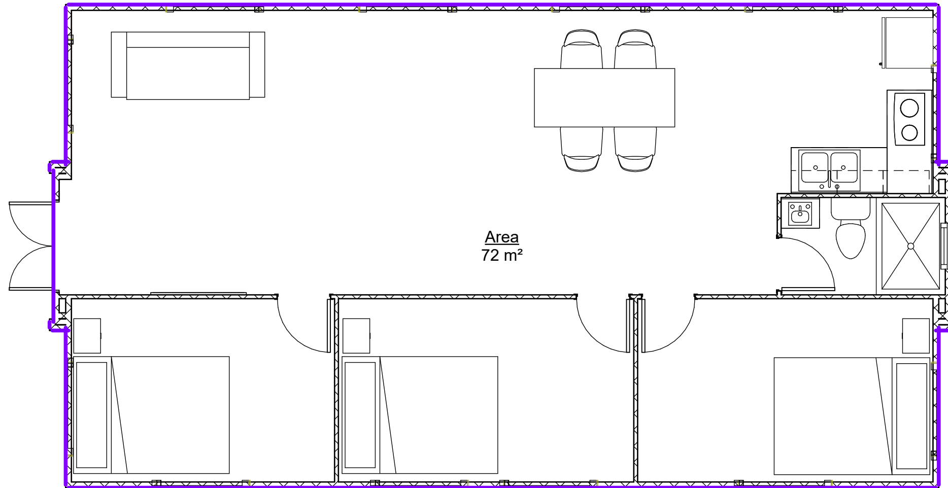
1 AREA PLAN 1 : 50
