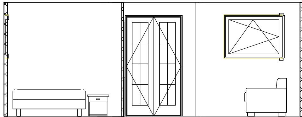
1 Section 1 1 : 50
