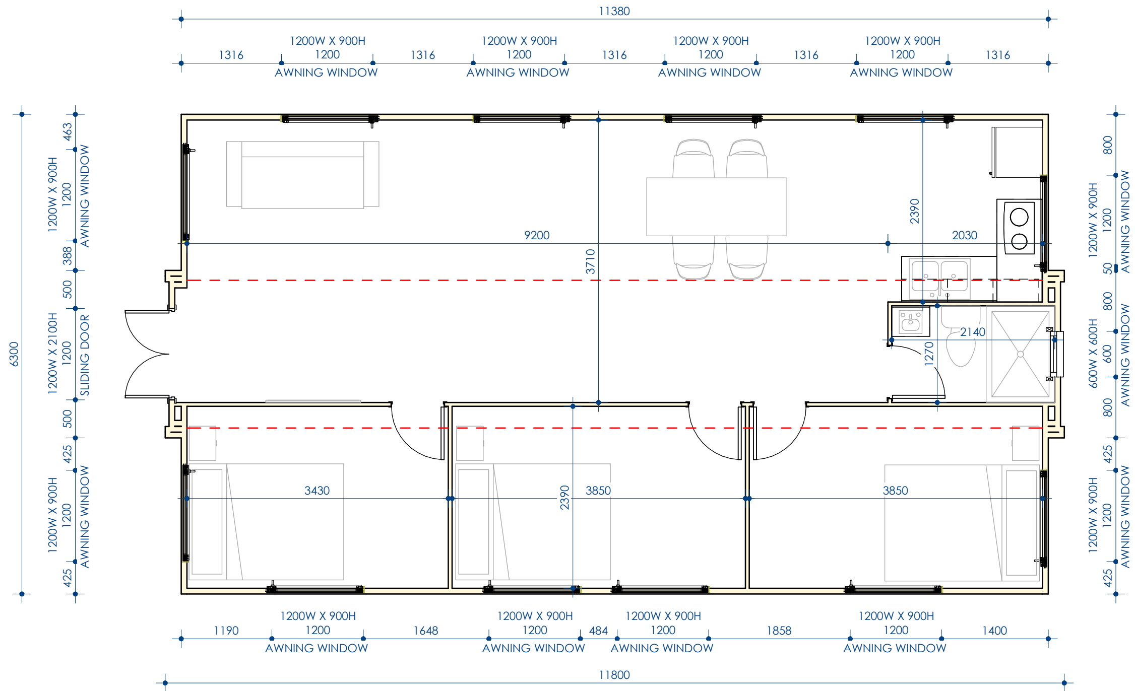
1 Level 1 1 : 50
