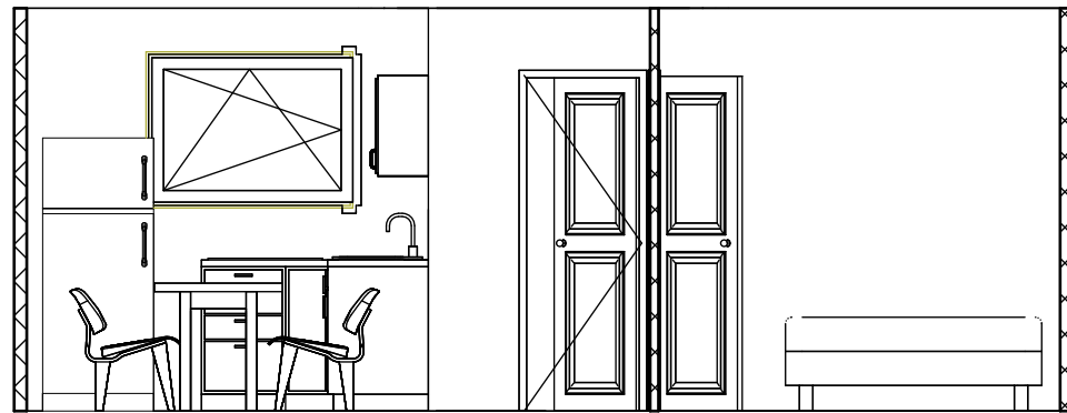
2 Section 2 1 : 50
