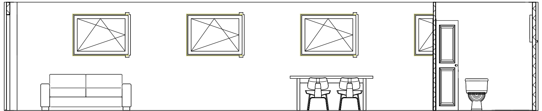
4 Section 4 1 : 50
