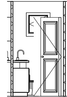
3 Section 3 1 : 50
