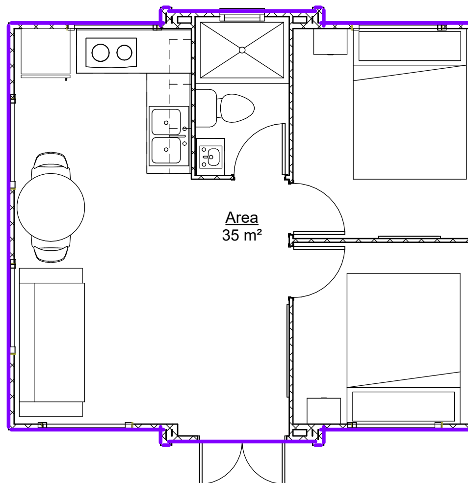
1 AREA PLAN 1 : 50
