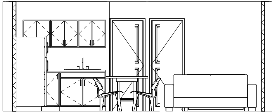
1 Section 1 1 : 50
