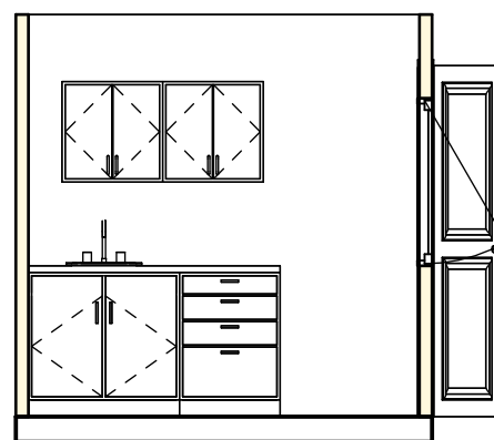
3 Section 3 1 : 50
