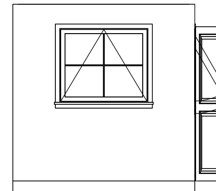
4 West 1 : 50
