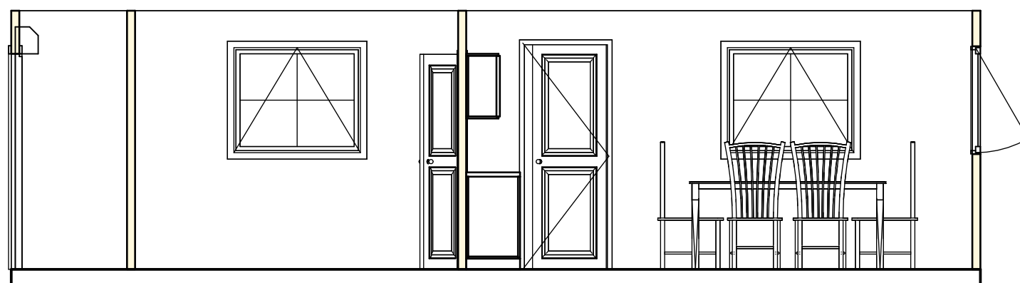
2 Section 2 1 : 50
