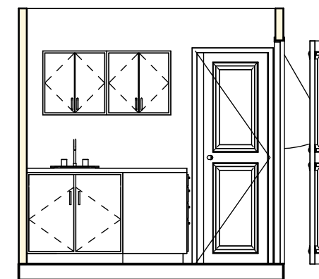
3 Section 3 1 : 50
