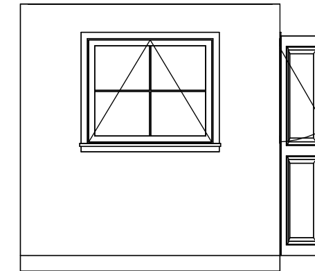
4 West 1 : 50
